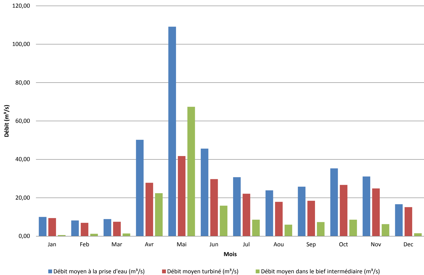
Figure A-4 : Distribution des débits mensuels moyens pour le bief intermédiaire du projet HCSJ
